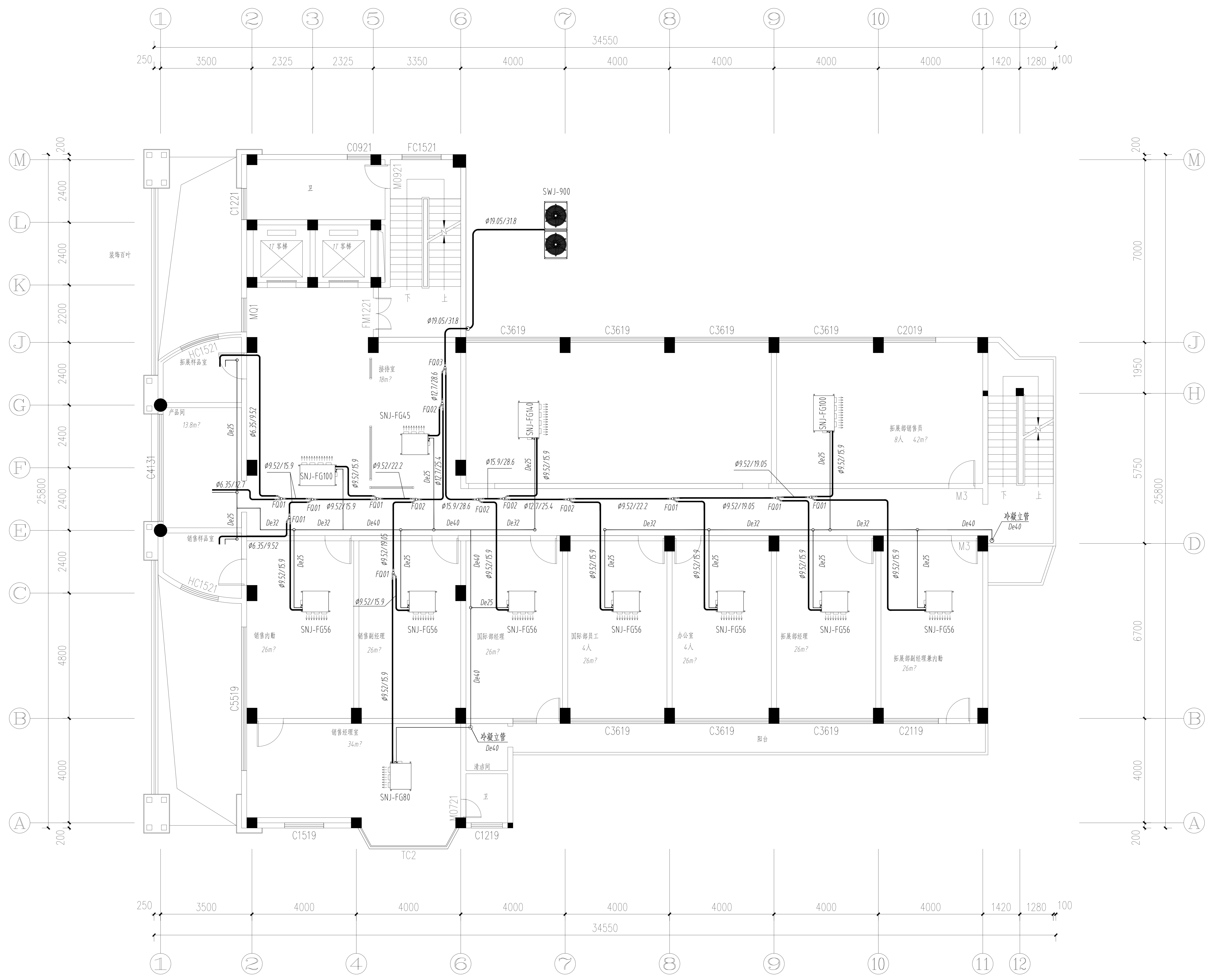
二层空调管道平面图 1:100
